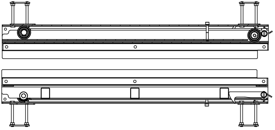
PRZEKRÓJ B-B SKALA 1 : 10
